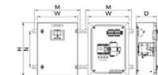
ATS Panel 63A
