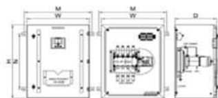
ATS Panel 250A
